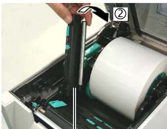
Obere Sensoreinheit
