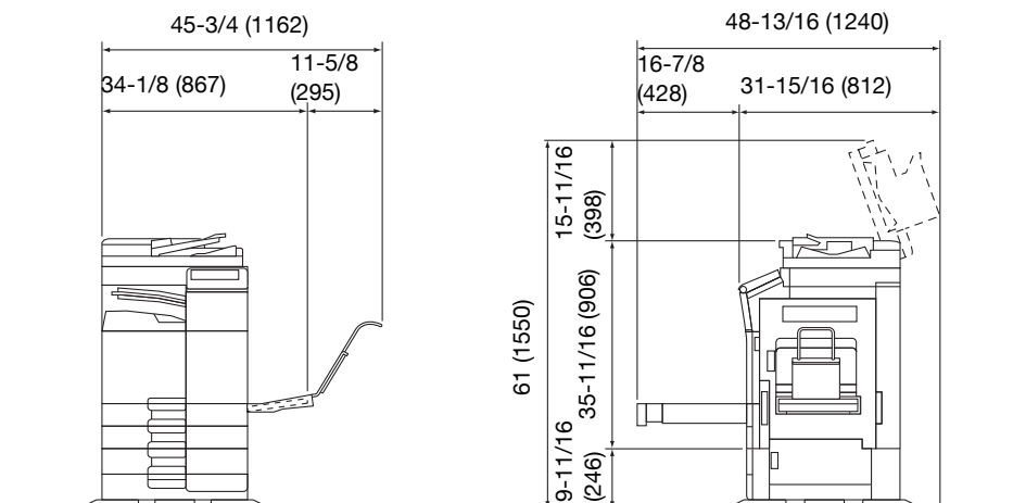
ineo 224e/284e/364e + DF-624 + PC-210 + JS-506 + MK-730
