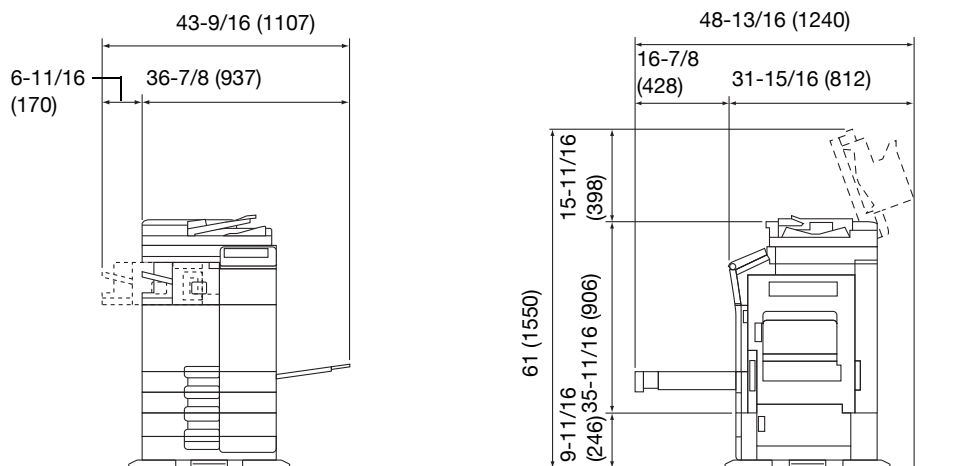
ineo 224e/284e/364e + DF-624 + PC-210 + FS-533
