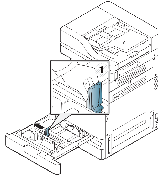
1 Papierbreitenführung
